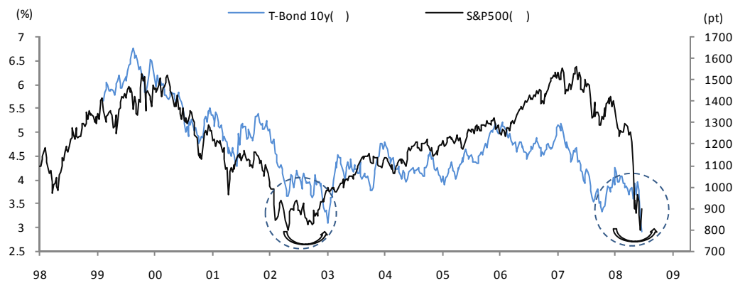
[ 4] 10 S&P500
