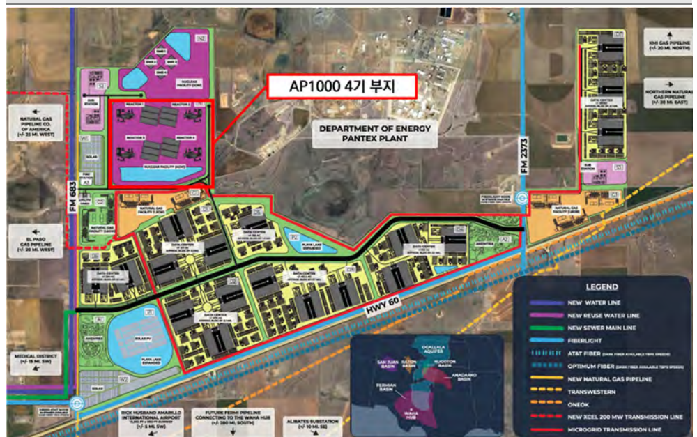
그림 100. 페르미 아메리카 마타도어 캠퍼스 AP1000 부지
