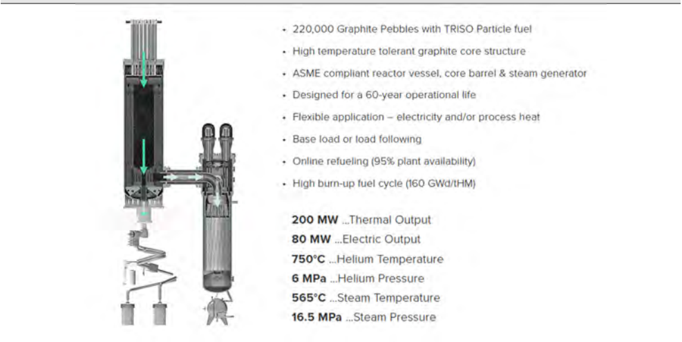
그림 110. X-에너지 Xe-100 모듈
