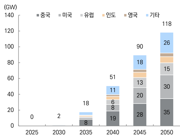
그림 118. IEA 지역별 SMR 원자로 증설 전망 (APS 기준)
