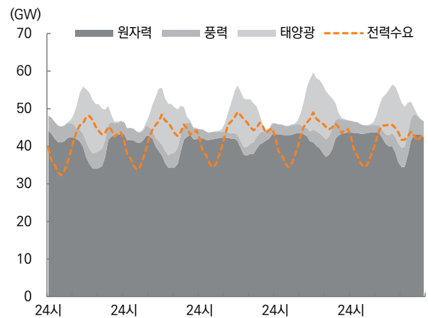
그림 81. 프랑스 25년 8월 전력 수요 및 발전 믹스
