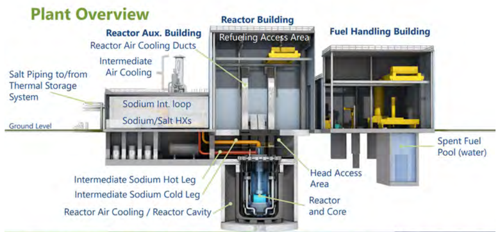
그림 109. 테라파워 Natrium 모듈
