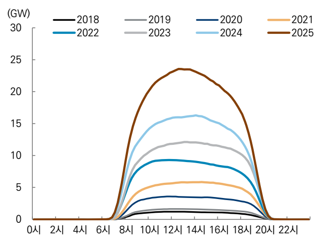
그림 40. 미국 PJM 시간별 태양광 발전량 추이
