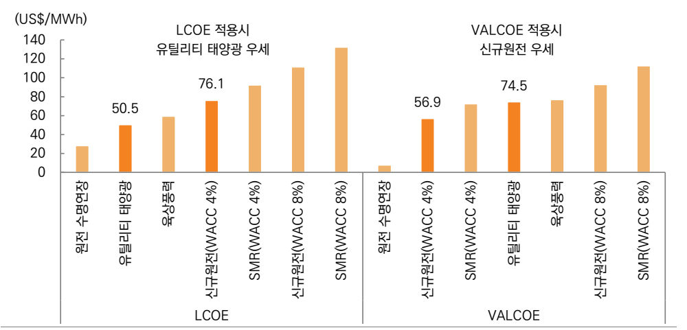
그림 56. APS 시나리오 유럽 에너지원별 LCOE vs VALCOE
