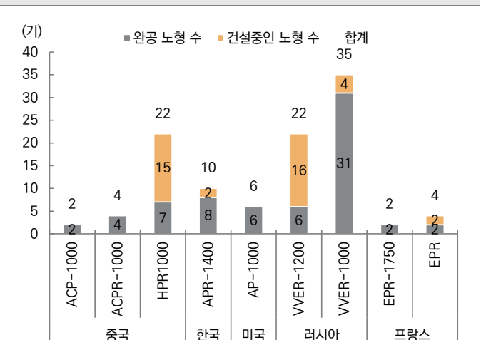
그림 93. 주요 원자로 공급사별 운영 및 건설 노형 수
