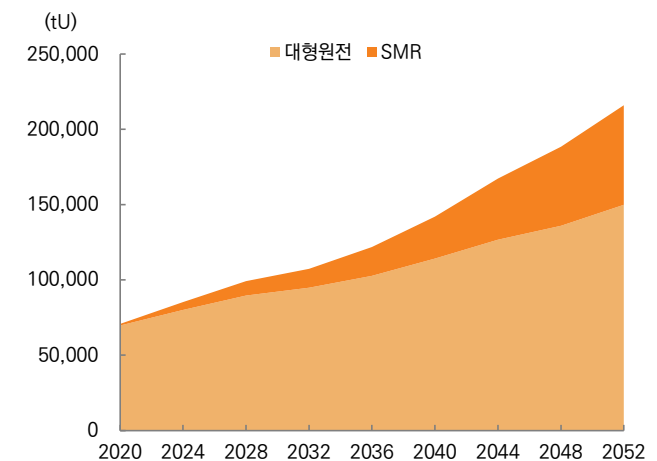
그림 128. 글로벌 원자력 발전용량에 따른 우라늄 수요 전망
