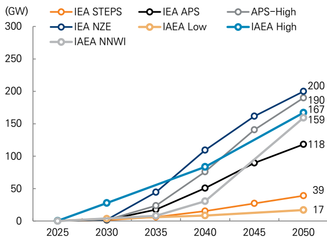
그림 75. 기관별 SMR 증설 전망
