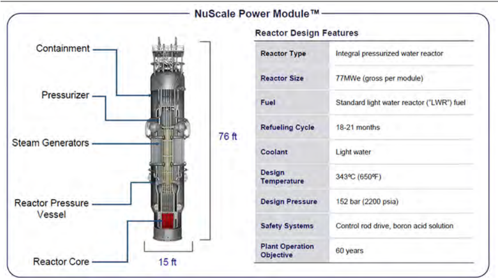
그림 108. 뉴스케일 파워 NPM 모듈
