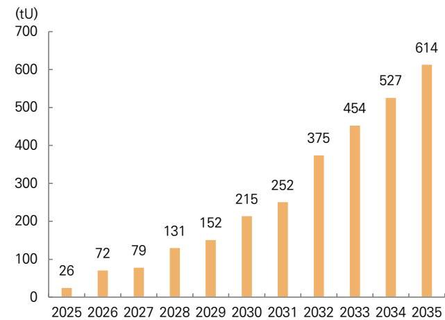
그림 132. 미국의 연간 HALEU 수요 추정치
