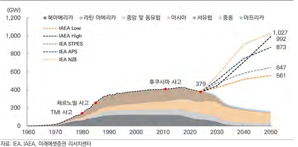
그림 91. 글로벌 시나리오별 원자력 발전소 용량 전망
