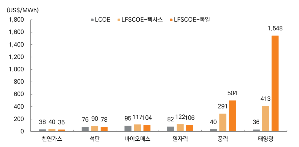
그림 53. 에너지원별 LCOE vs LFSCOE 비교
