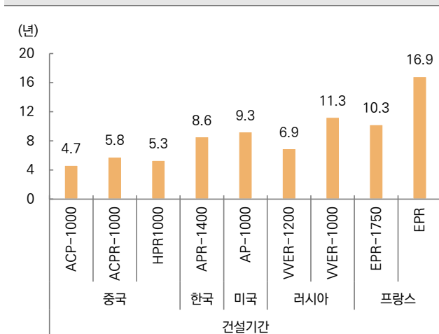
그림 92. 주요 원자로 공급사별 평균 건설 기간
