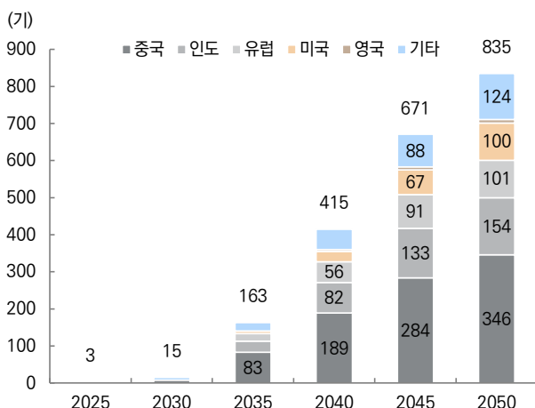
그림 77. IEA 지역별 SMR 원자로 설치수 추이 (APS 기준)
