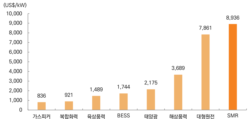
그림 198. EIA의 에너지원별 자본 비용 추정
