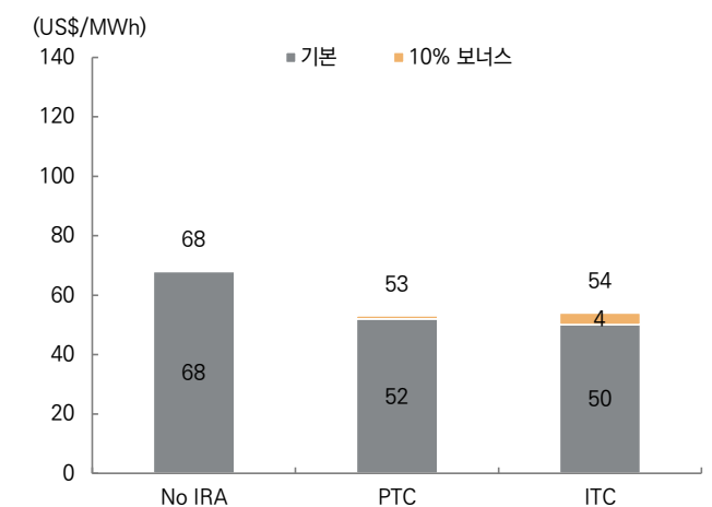
그림 230. IRA 세액공제에 따른 원자력 발전소 LCOE 변화
