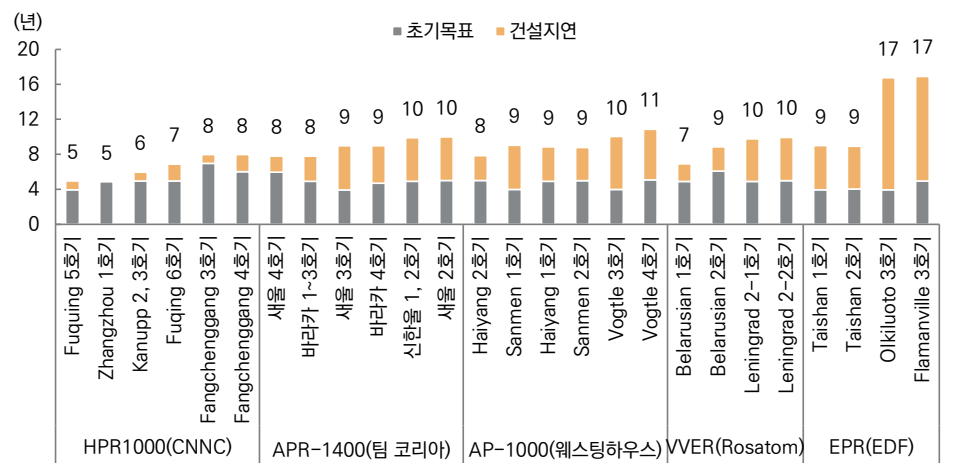
그림 95. 원자로 공급사 주요 노형별 원전 건설 기간
