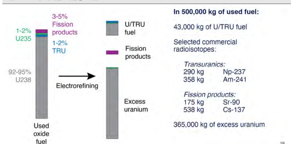
그림 224. 핵 폐기물 재활용 개념도
