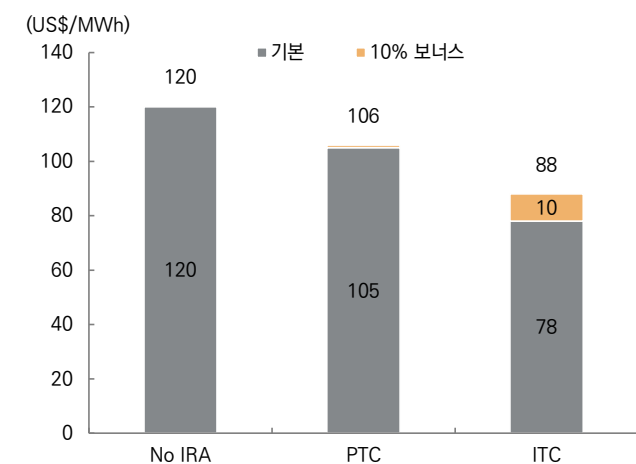
그림 229. IRA 세액공제에 따른 원자력 발전소 LCOE 변화
