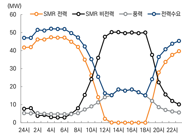
그림 80. SMR 탄력운전 활용방안
