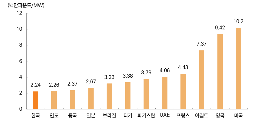
그림 97. 2000년 이후 국가별 원전 건설단가
