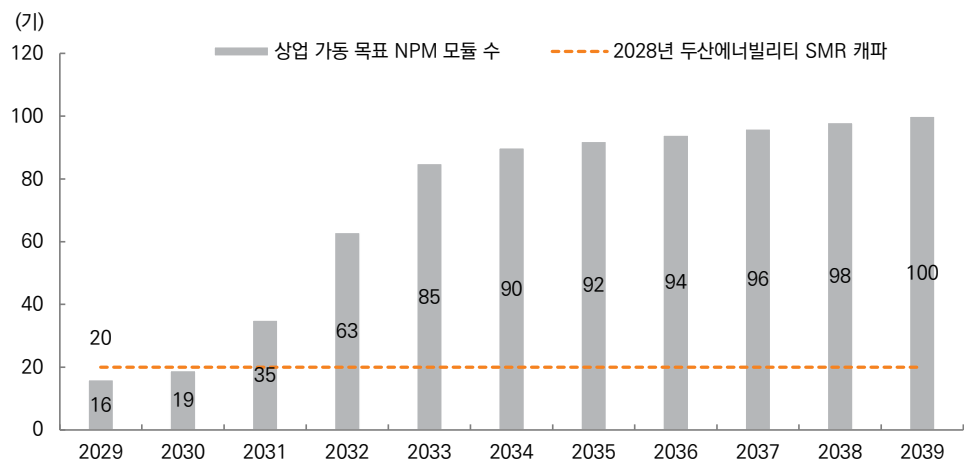
그림 202. 뉴스케일 파워 상업 가동 목표 NPM 모듈 수(2021년) vs 두산에너지빌리티 SMR 개파
