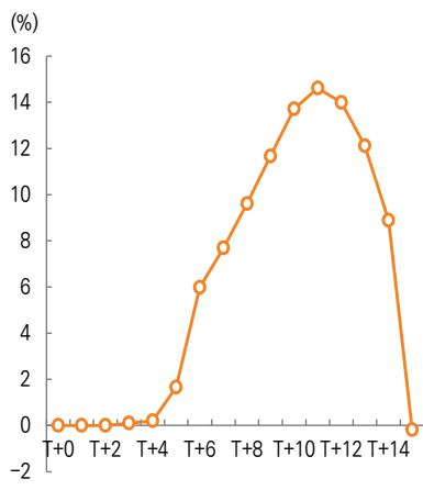
그림 29. 한전 KPS 수익 인식 흐름
