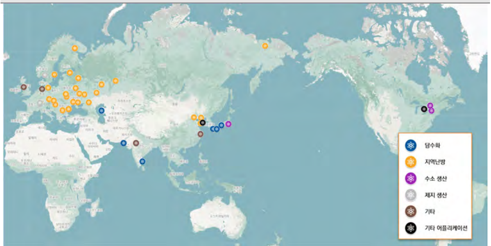
그림 82. 발전 외 원자력 활용 현황
