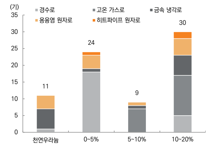
그림 216. SMR 노형별 필요 우라늄 농축도
