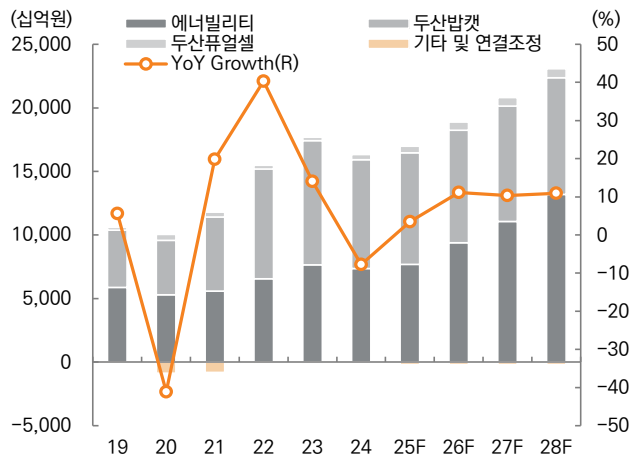
그림 148. 두산에너지빌리티 매출액 추이(연결)
