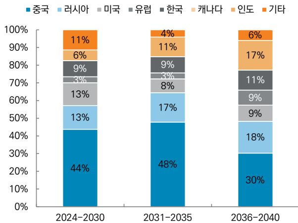
그림 115. 주요 원자로 수출 국가별 수주 비중 추정
