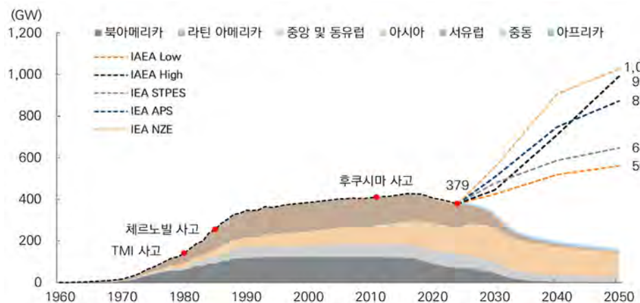
그림 35. 글로벌 시나리오별 원자력 발전소 용량 전망
