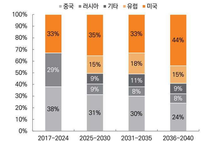
그림 121. IEA 전망 주요 원자로 수출 국가별 SMR 수주 비중
