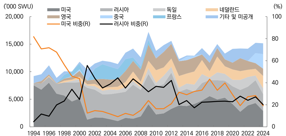
그림 134. 미국의 국가별 우라늄 농축설비 대여 추이
