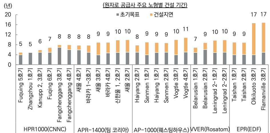
그림 14. 납기 준수 능력을 바탕으로 글로벌 원전 수주를 확보할 수 있을 것으로 기대
