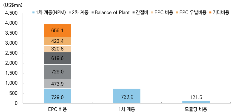
그림 197. EIA SMR 발전소 자본비용 추산
