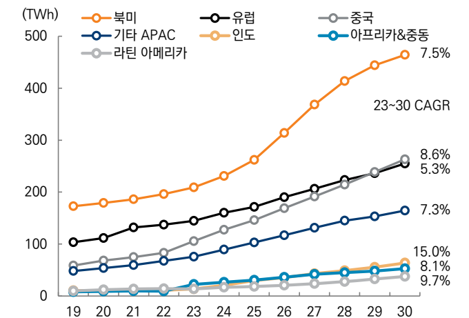
그림 60. 데이터센터 증설에 따른 지역별 전력 수요
