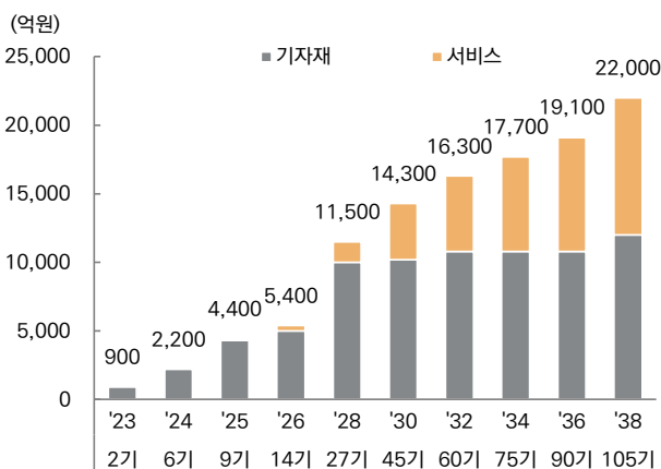
그림 165. 두산에너지빌리티 가스터빈 사업 매출 전망
