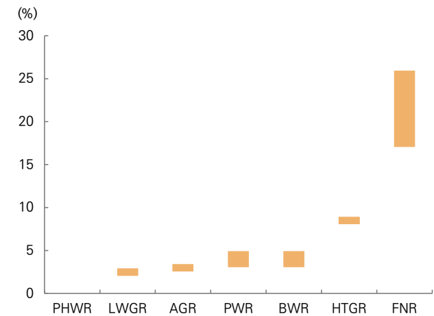
그림 131. 원자노형별 요구되는 우라늄 농축 비율
