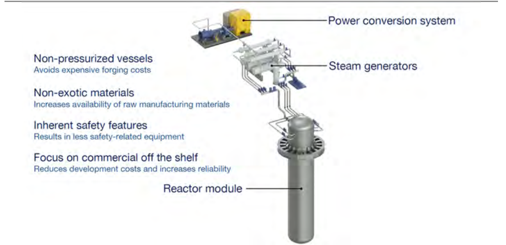
그림 227. Aurora 모듈 발전 구조
