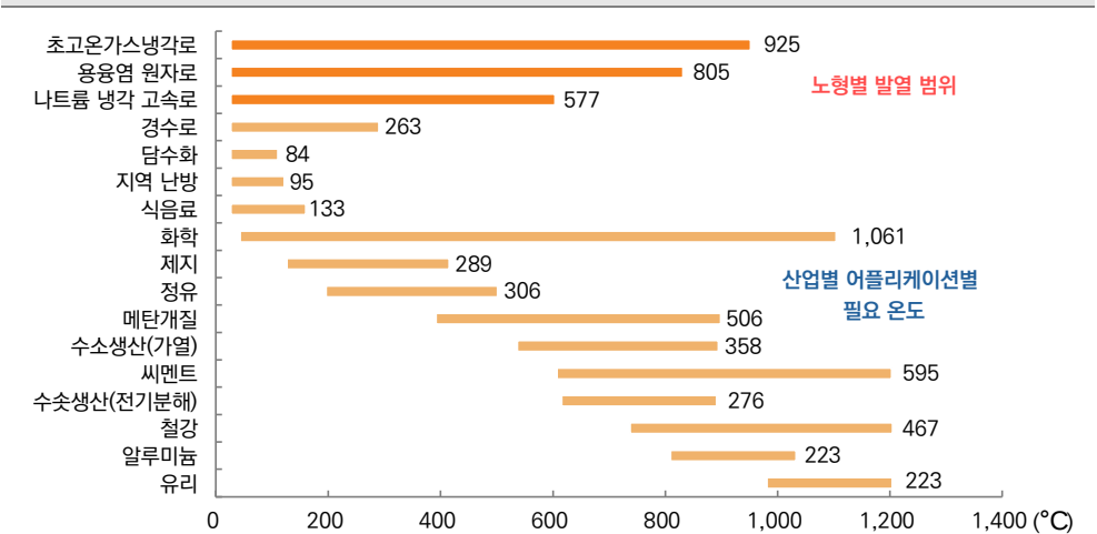
그림 83. 산업용 어플리케이션별 필요 온도 vs 노형별 발열 범위
