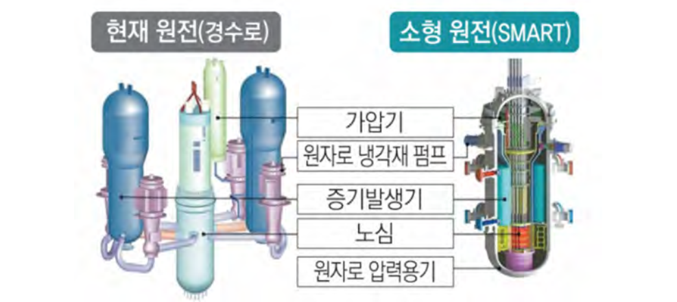
그림 79. 대형원전과 SMR(SMART) 비교
