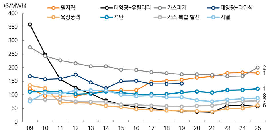
그림 51. 글로벌 에너지원별 LCOE 추이
