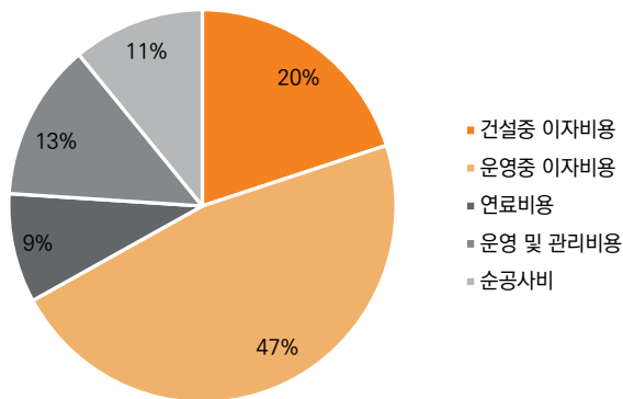
그림 85. 원자력 발전소 LCOE 구성
