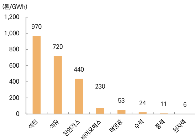
그림 61. 주요 에너지원별 탄소 배출량
