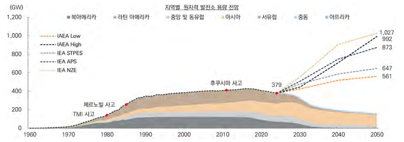
그림 2. 노후화와 인허가 만료에 따른 발전소 폐쇄를 고려 시 약 555GW의 원전 증설 필요
