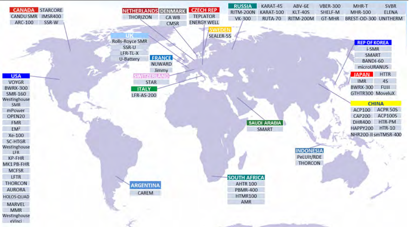
그림 105. 국가별 SMR 개발 현황
