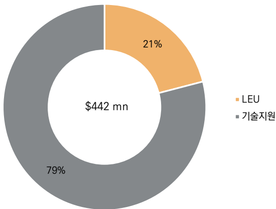
그림 139. 센트리스 에너지 사업부문별 매출 비중 그림 140. 센트리스 에너지 주요 사업 부문
