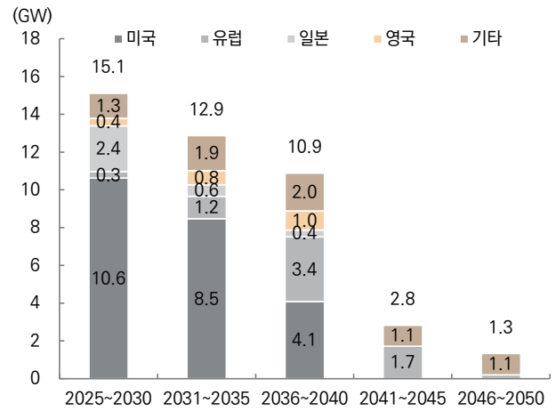
그림 114. 미국-웨스팅하우스 지역별 신규 증설 전망
