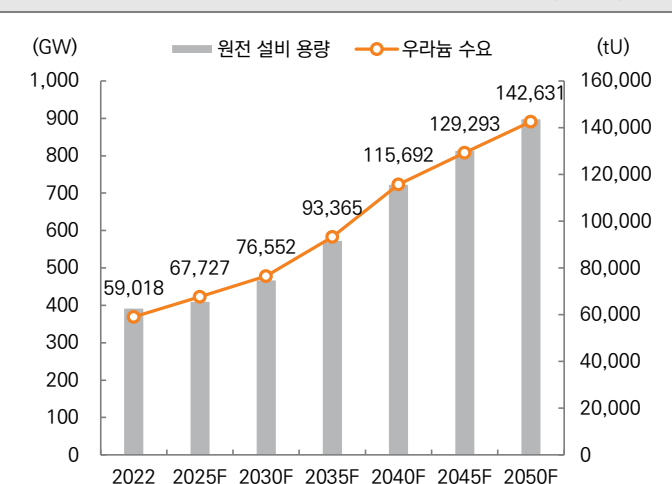
그림 126. 글로벌 원전 설비용량 및 우라늄 수요 전망 (고수요)
