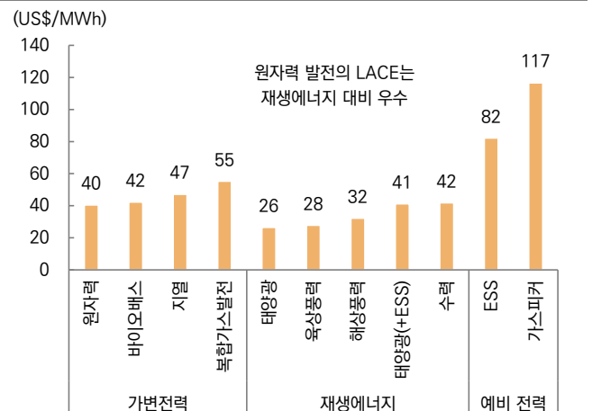
그림 58. 미국 에너지원별 LACE 비교
