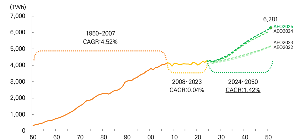
그림 84. 미국 전력 수요 추이 및 전망
