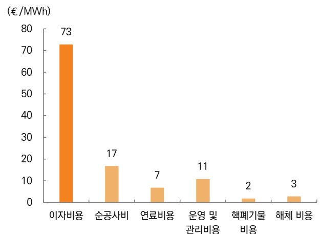
그림 102. Hinkley Point C MWh당 항목별 비용
