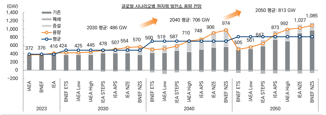
그림 1. 에너지 전망 기관들은 2050년까지 평균적으로 약 813GW의 원자력 발전용량을 전망
