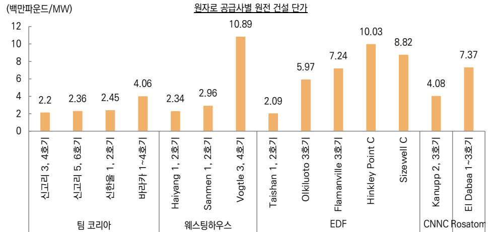
그림 13. 팀 코리아는 경쟁사 대비 건설단가가 낮으며
