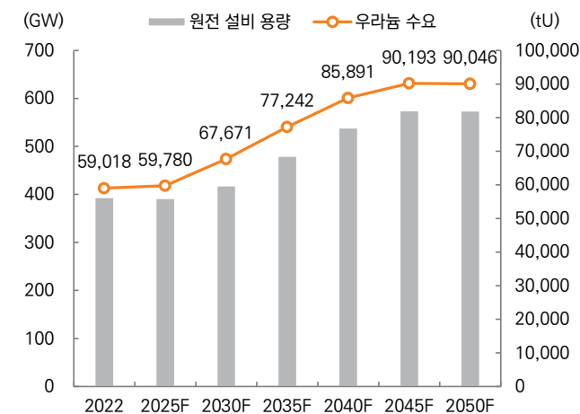
그림 188. 글로벌 원전 설비용량 및 우라늄 수요 전망 (저수요)
