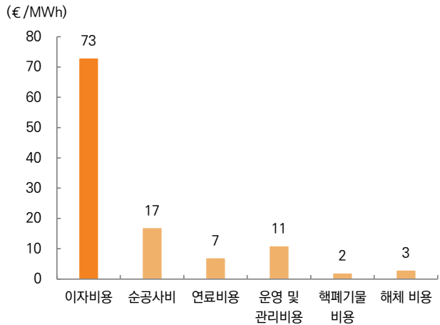
그림 86. Hinkley Point C MWh당 항목별 비용
