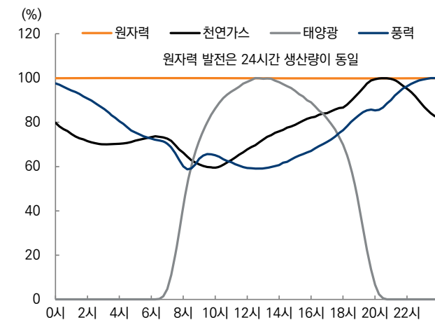
그림 43. 에너지원별 일일 전력 생산량 추이
