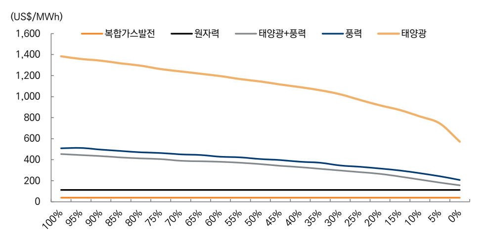
그림 54. 에너지 저장장치 가격에 따른 에너지원별 LFSCOE 비교
