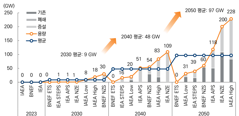
그림 117. 글로벌 시나리오별 SMR 발전소 용량 전망
