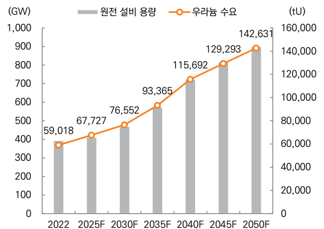
그림 189. 글로벌 원전 설비용량 및 우라늄 수요 전망 (고수요)
