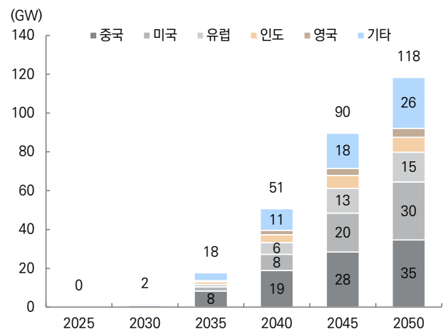
그림 76. IEA 지역별 SMR 원자로 증설 전망 (APS 기준)
