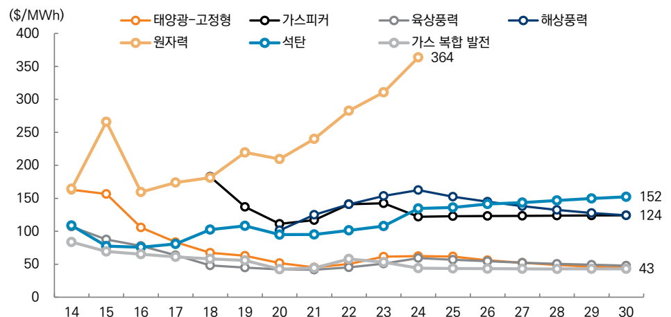
그림 52. 미국 에너지원별 LCOE 추이 및 전망
