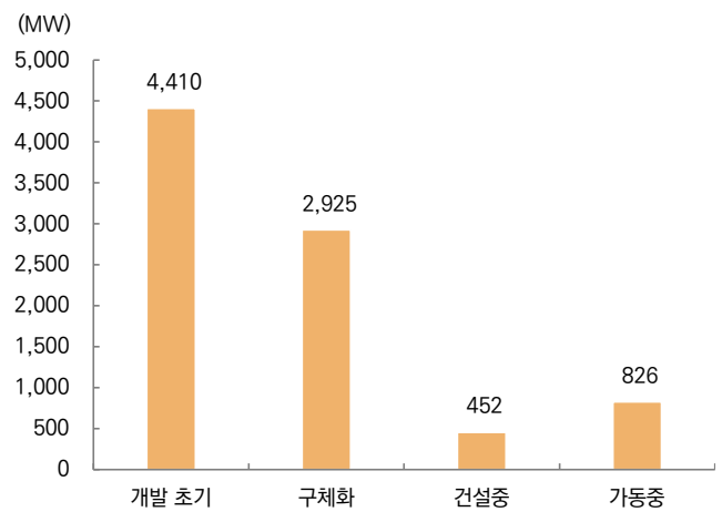
그림 104. SMR 개발 현황
