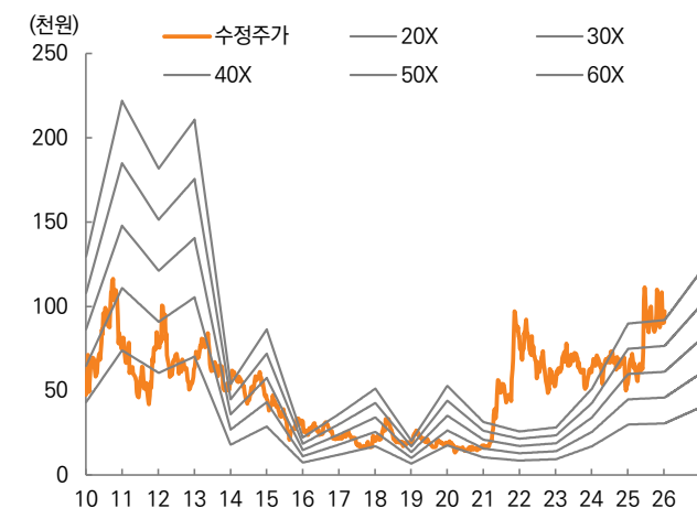
그림 170. 한전기술 12MF PER 밴드 차트
