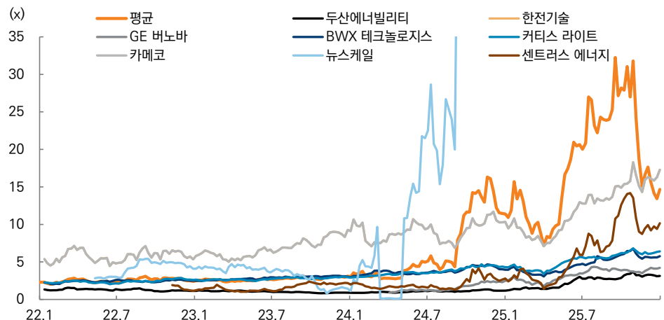
그림 19. 원전 및 우라늄 기업 EV/SALES 멀티플 추이
