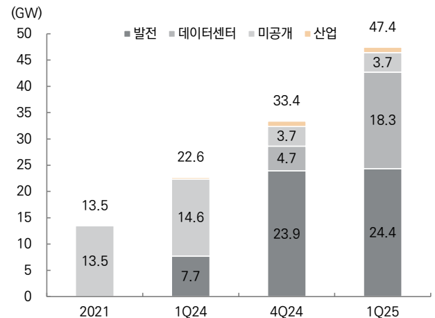
그림 70. 미국 어플리케이션별 SMR 파이프라인 현황
