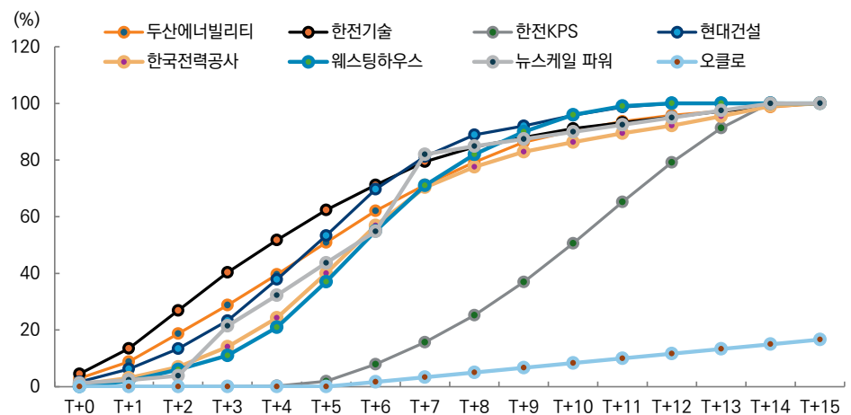
그림 22. 원전 사업 개시 후 연도별 누적 진행률 추이
