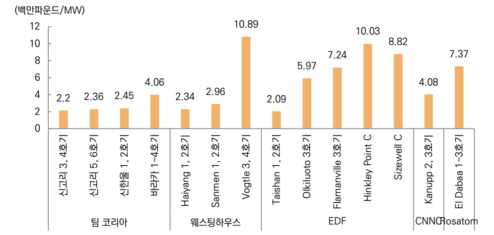
그림 96. 원자로 공급사별 원전 건설단가
