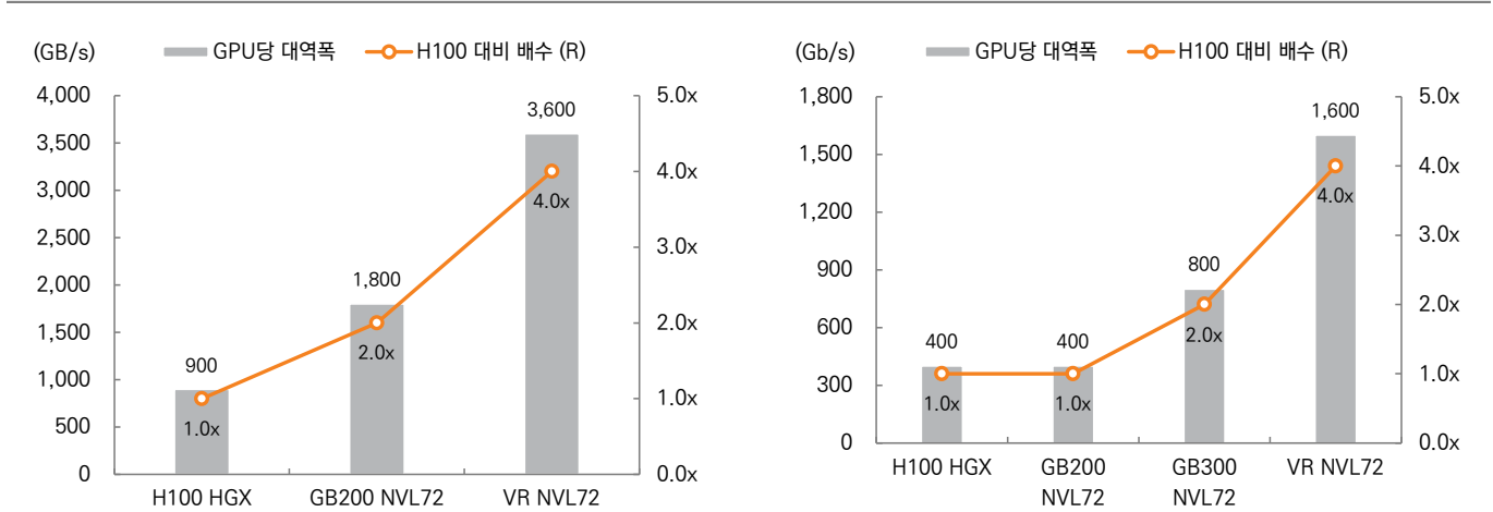
그림 23. GPU당 NVLink scale-up 대역폭 그림 24. GPU당 scale-out 대역폭
