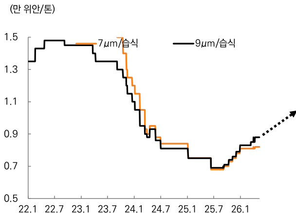
그림 80. 중국 습식 분리막 가격 추이 → 우상향 지속 예상
