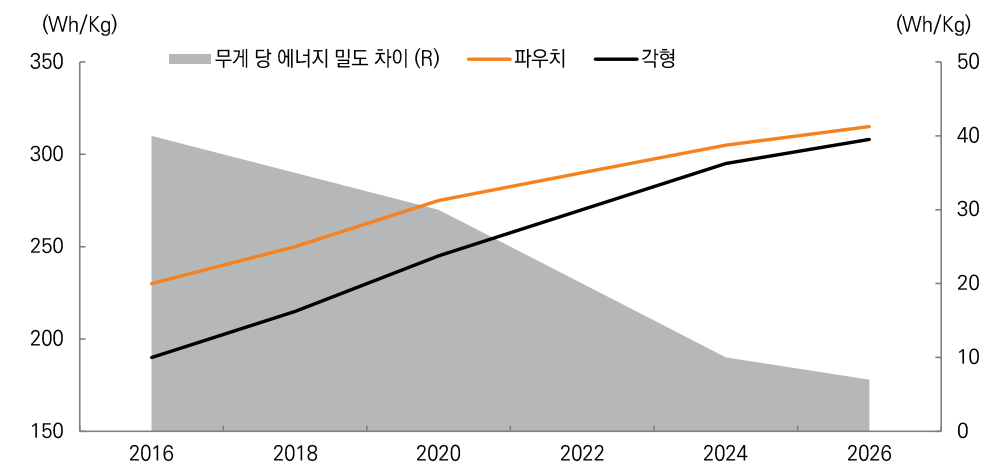
그림 59. 각형 배터리, 파우치와 무게 당 에너지 밀도 차이 축소
