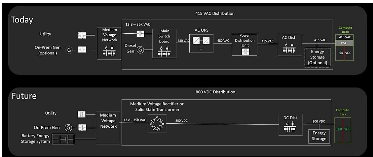
그림 32. 데이터센터 전력 분배 구조 전환 (415V AC → 800V DC)
