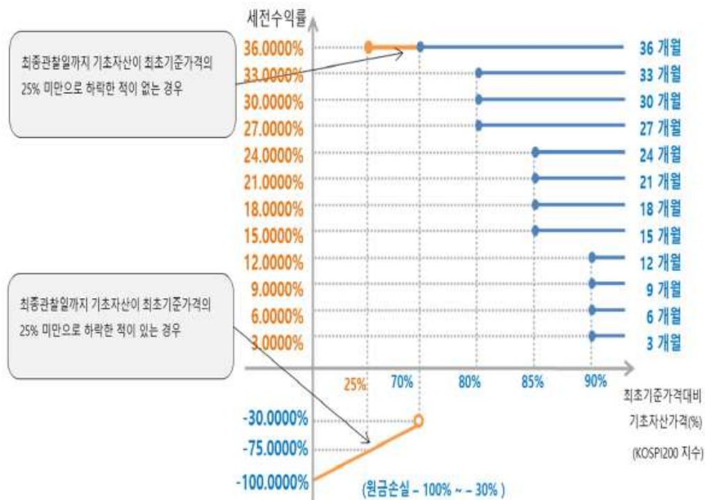
미래에셋증권 제38024회 (예상 손익구조 그래프)
