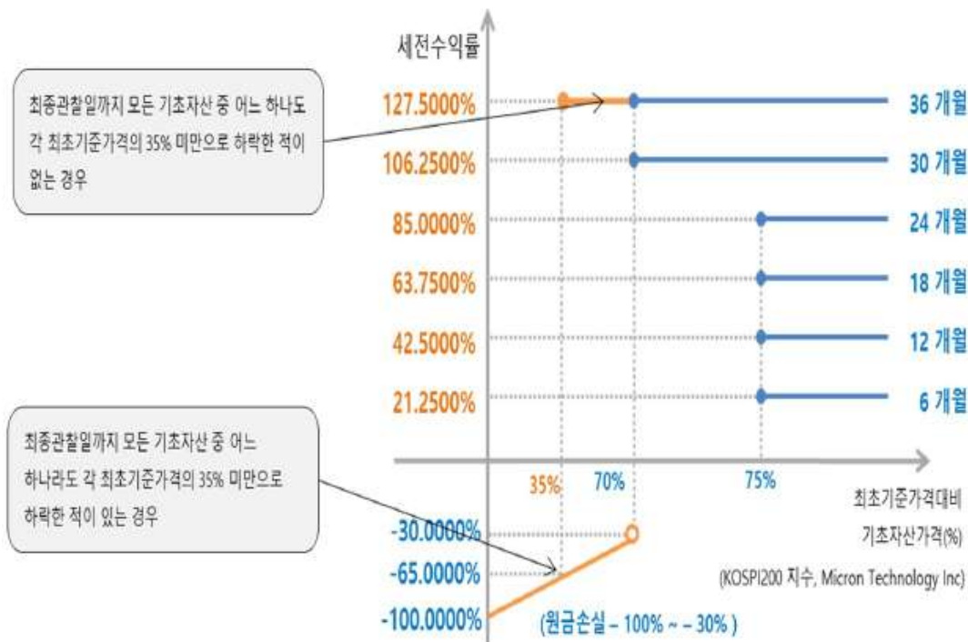
미래에셋증권 제38023회 (예상 손익구조 그래프)
