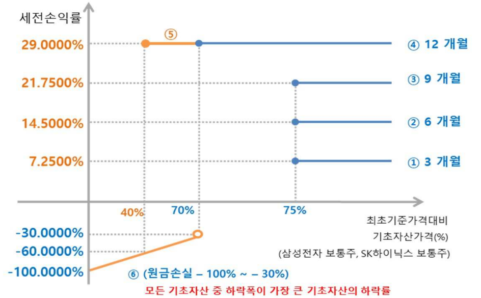
■ 손익구조 그래프
